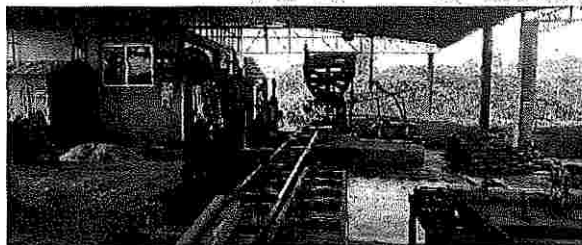
Torre de aserrio principal con carro
