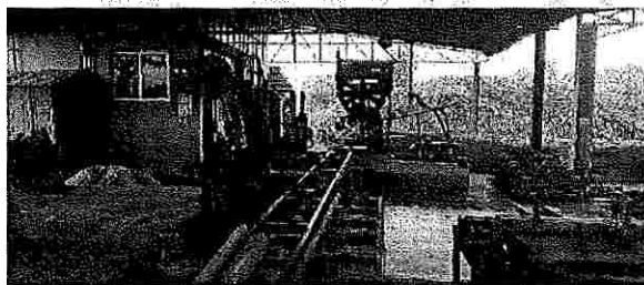
Torre de aserrío principal con carro
