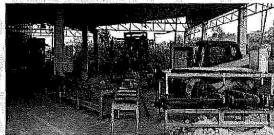
Torre de aserrío principal con carro y trimmer
